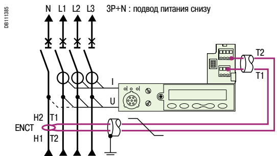
Внешний трансформатор тока нейтрали: ENCT
