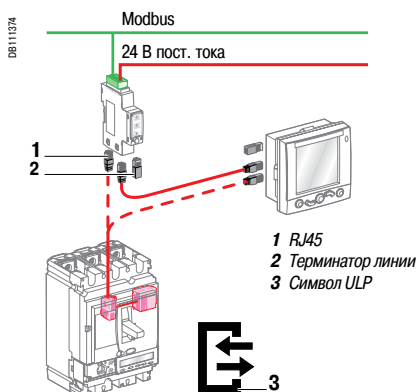
Соединительная система ULP
