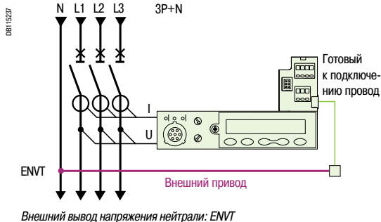
Внешний вывод напряжения нейтрали: ENVT
