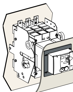
Стандартная рамка передней панели с мотор-редуктором
